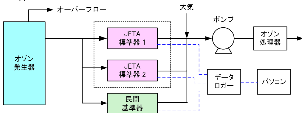
図2 オゾン濃度値付けの流路系統図
