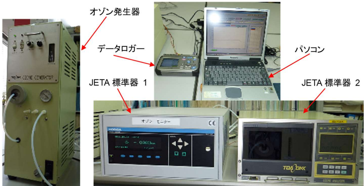
図3 装置外観写真
